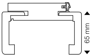
Kantenausführung eckig
